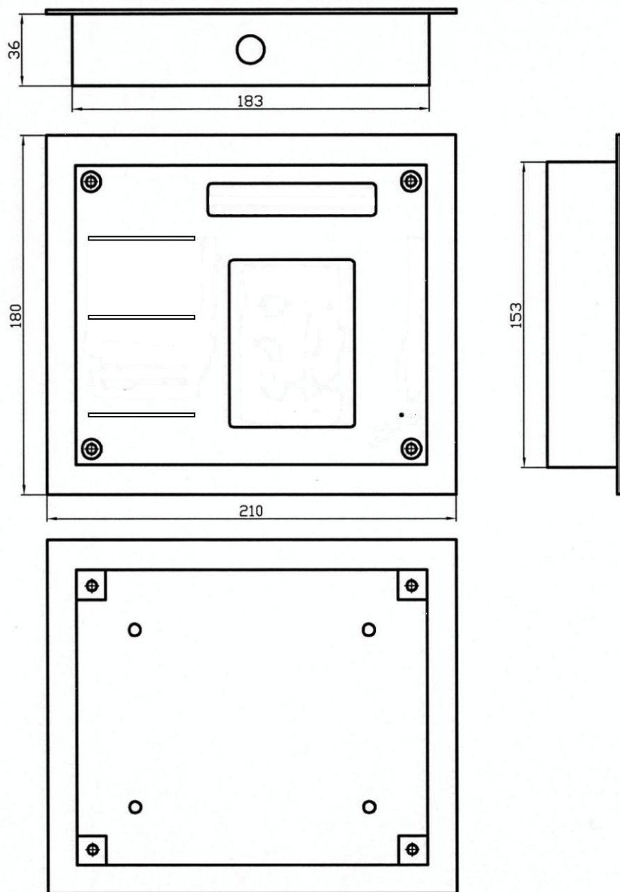
Рис.1 – Размеры корпуса
