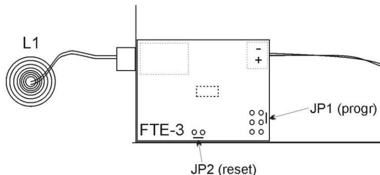
Рис.2 Программирование RFID фильтра FTE-3
