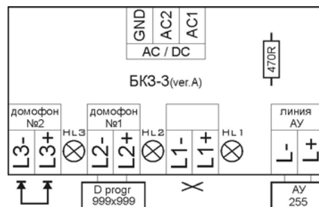
Рис.2 «Программирование»
