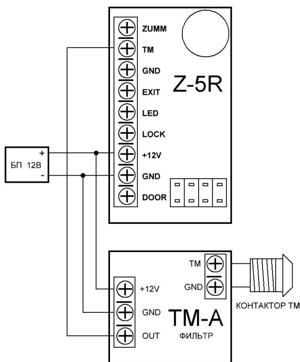
Подключение фильтра TM-A к контроллеру Z-5R
