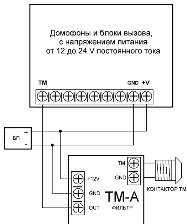
Подключение фильтра TM-A к домофону
